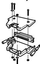
F377A body . . . 1
